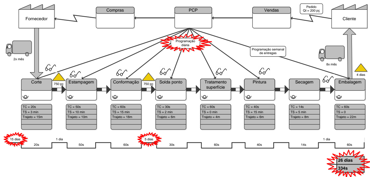
Figura 4 – Mapa do fluxo de valor atual
