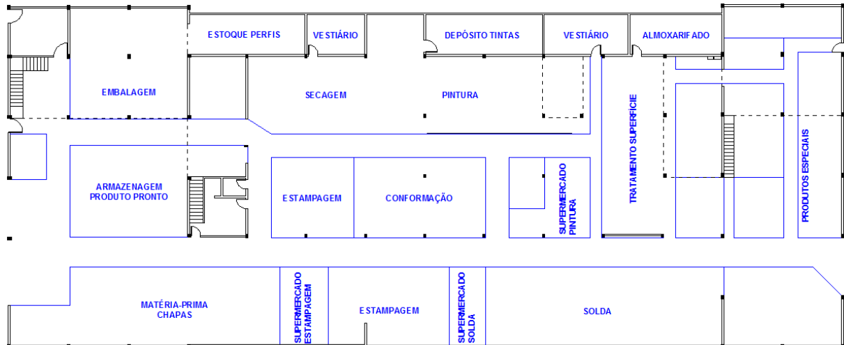
Figura 6 – Divisão setorial no layout proposto
