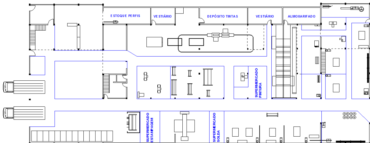
Figura 7 – Posicionamento das máquinas no layout proposto
