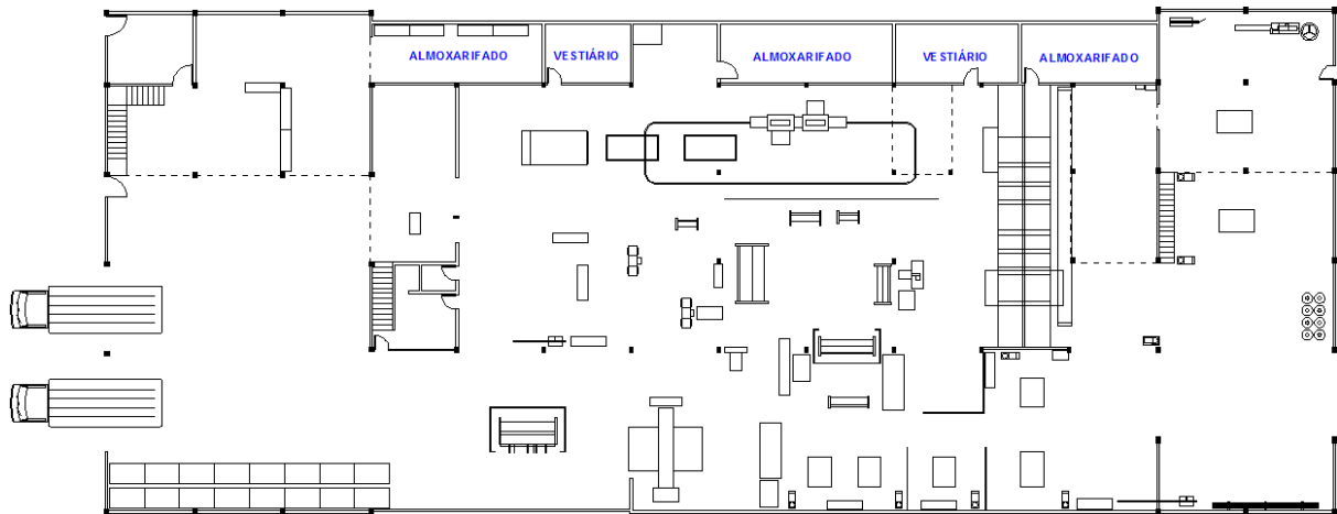
Figura 2 – Layout atual da empresa
